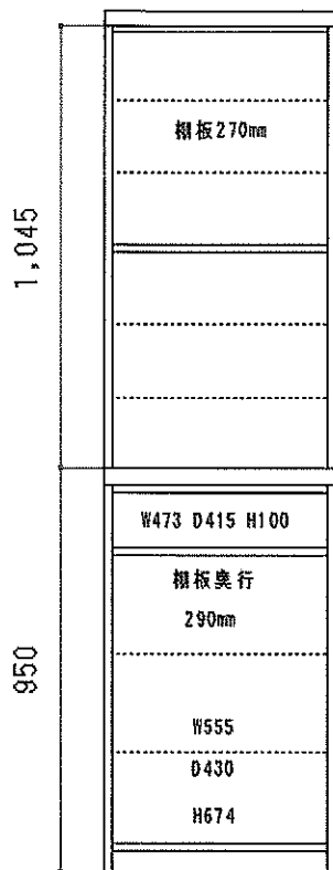
外寸: 60DB W600 D480 H2030
