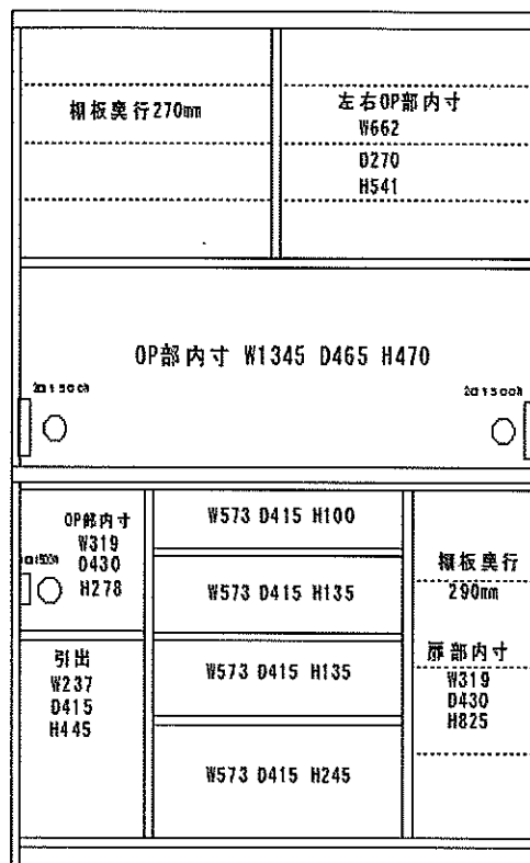
外寸: 1400P W1390 D480 H2030
